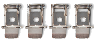
UCHWYT DO KARTON-GIPS DO PANELI O WYMIARACH 60X60
